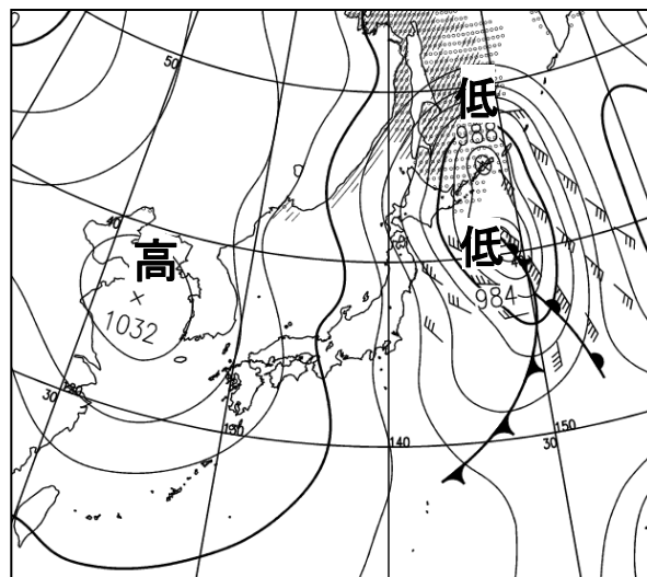
予想天気図 3月6日9時
