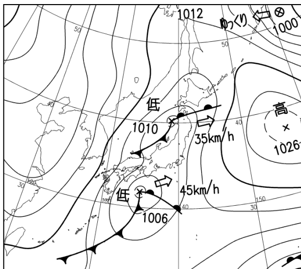
実況天気図 3月5日12時
