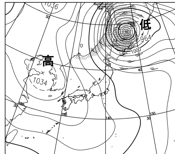
予想天気図 3月7日9時
